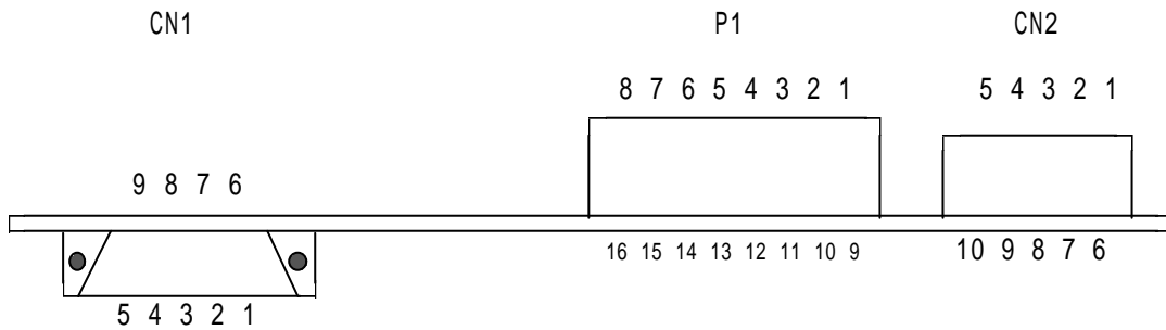
コネクタから見たピン番配置
