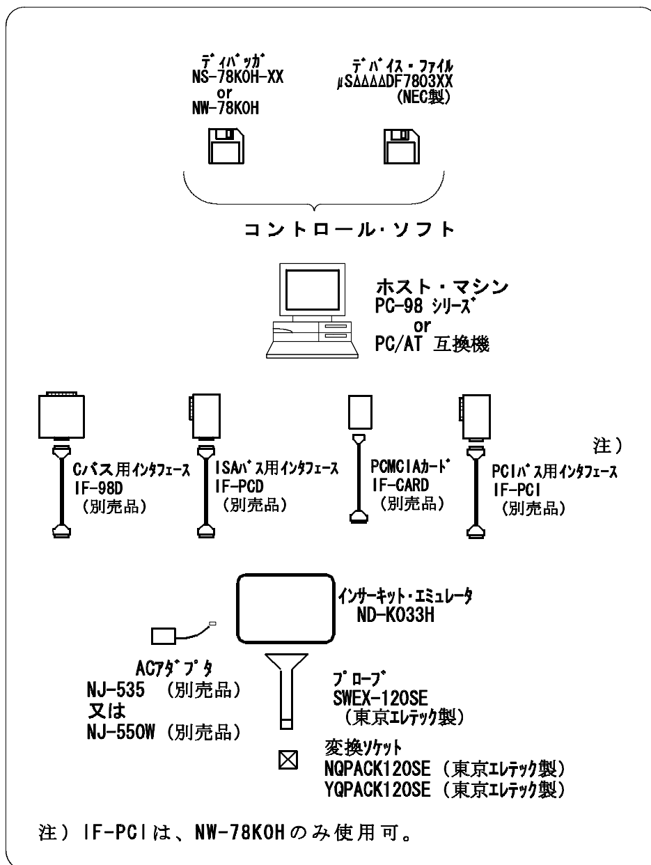
《ASMIS ND-K033H のシステム構成》
