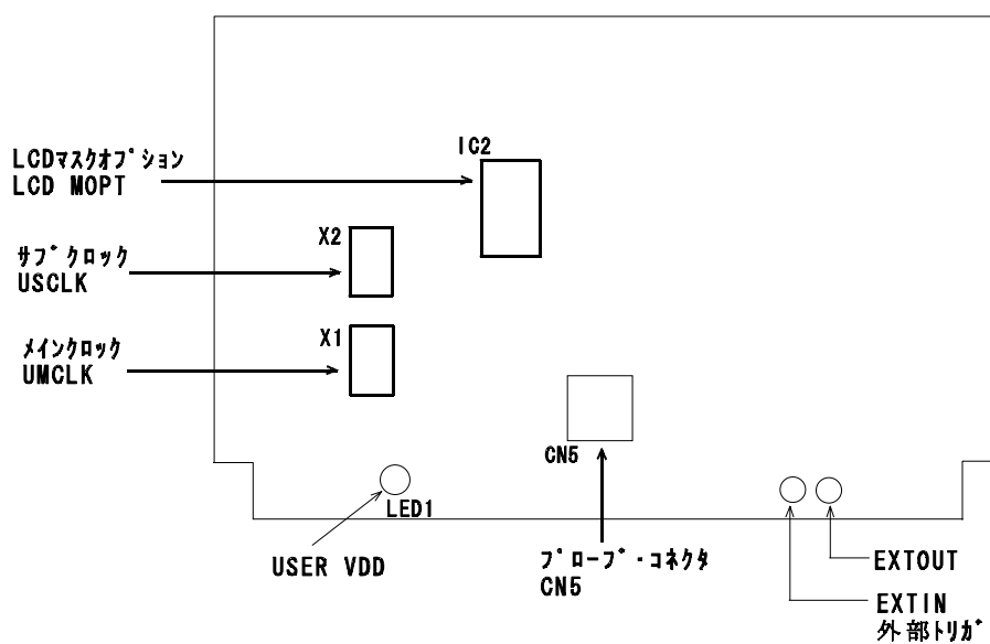
( b ) エミュレーション・ボード (G-780338 EM1 Board)
