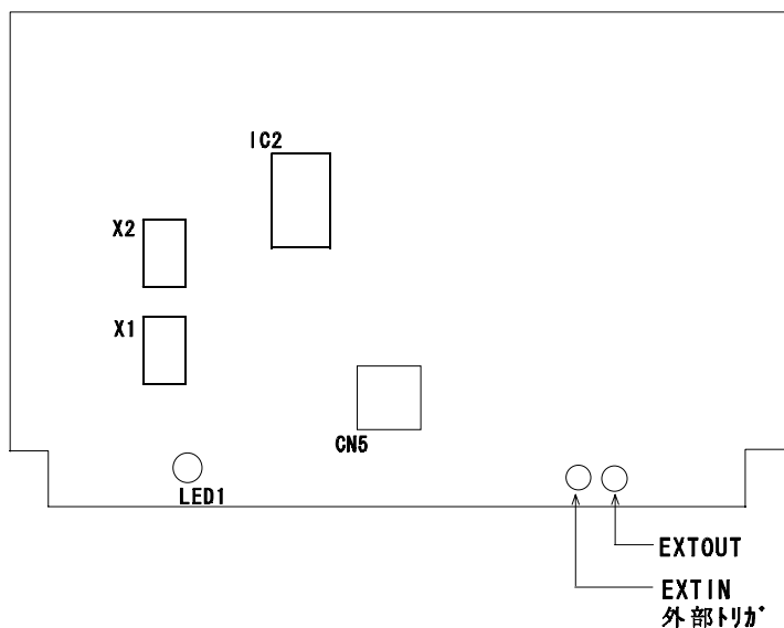
《 G-780338 EM1 Board 》
