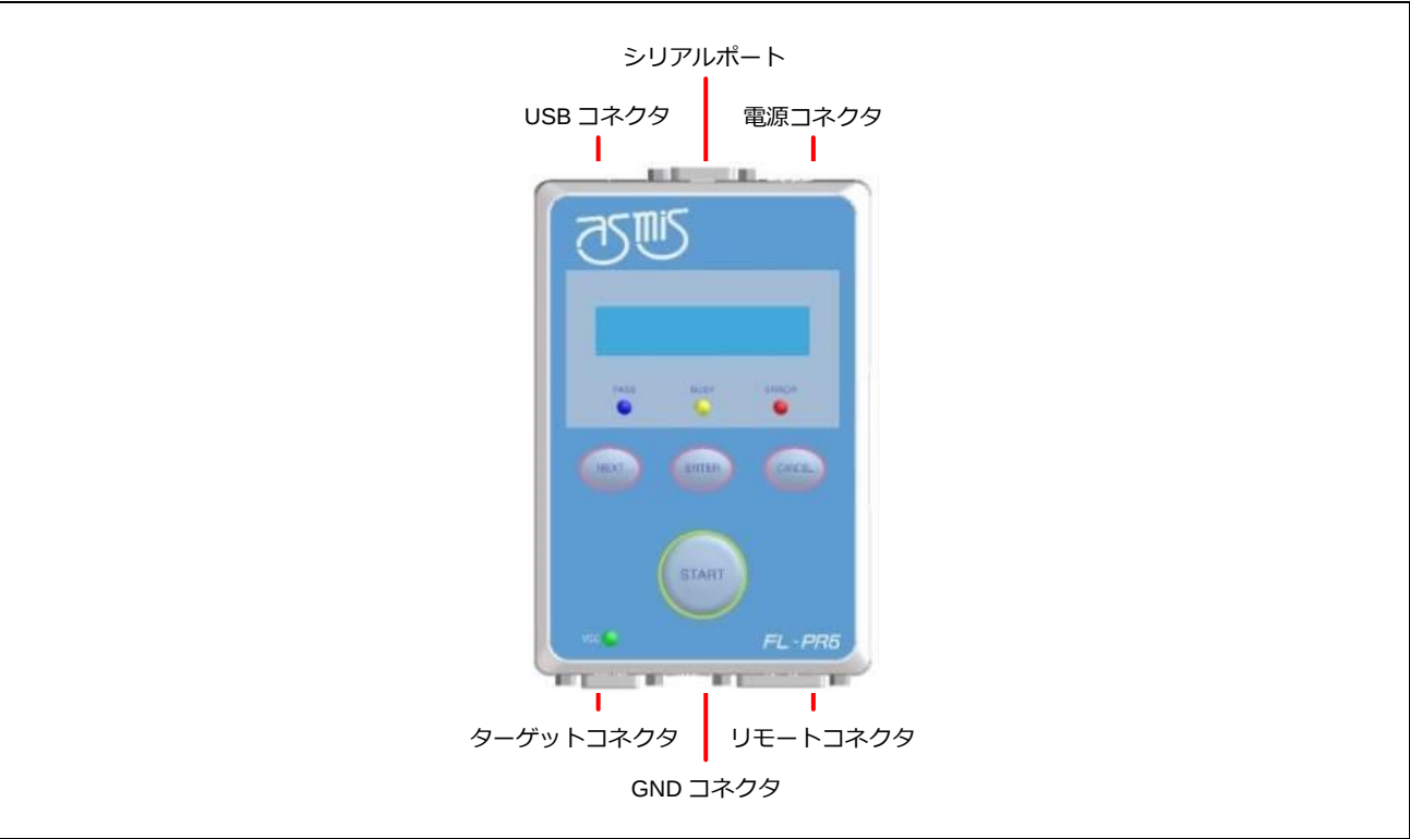
図 2.2 FP6 上面 <コネクタ>
