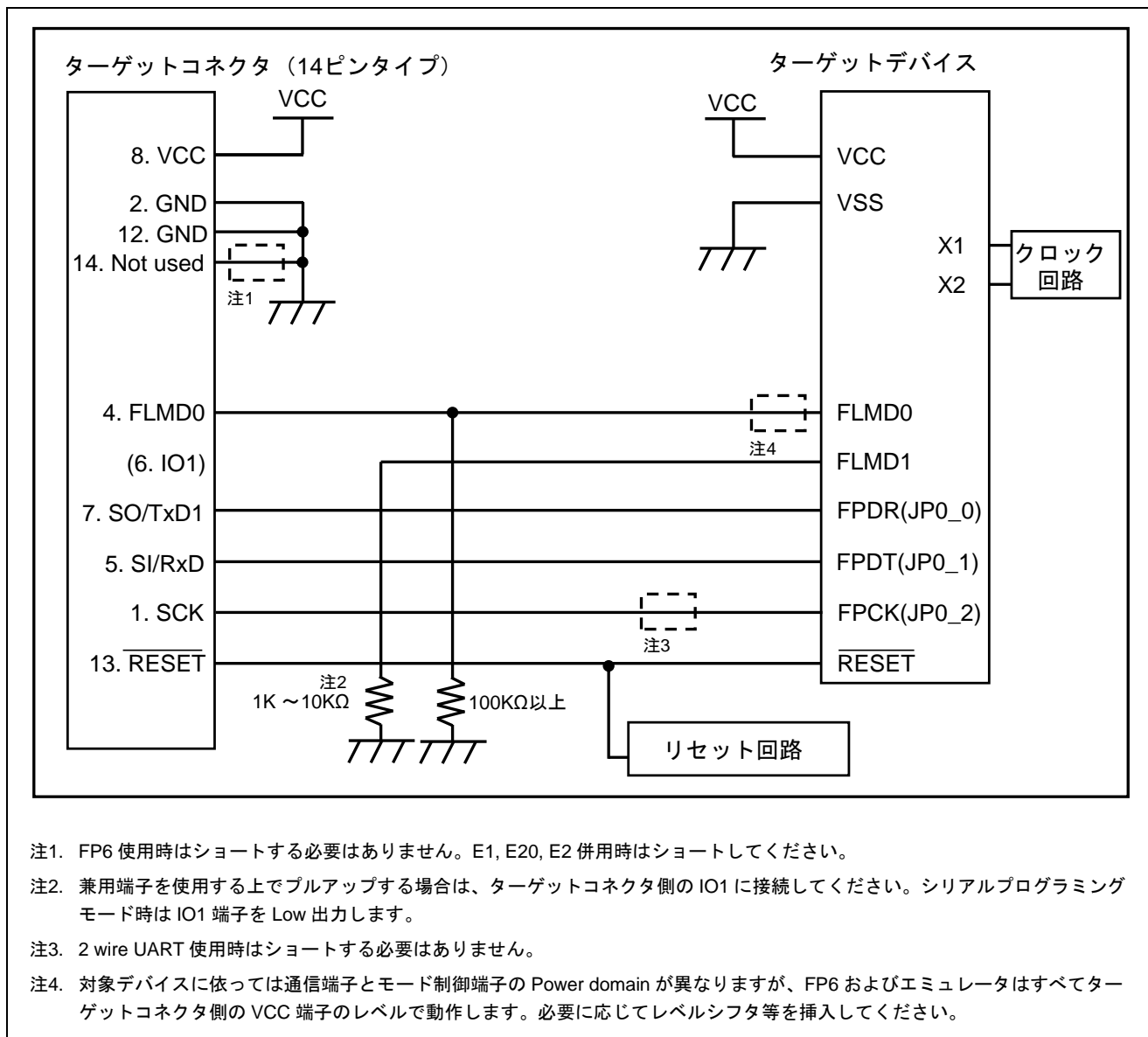
図 3.9 2 wire UART または CSI (RH850 ファミリ) の回路例 (RH850/F1x の回路例)
