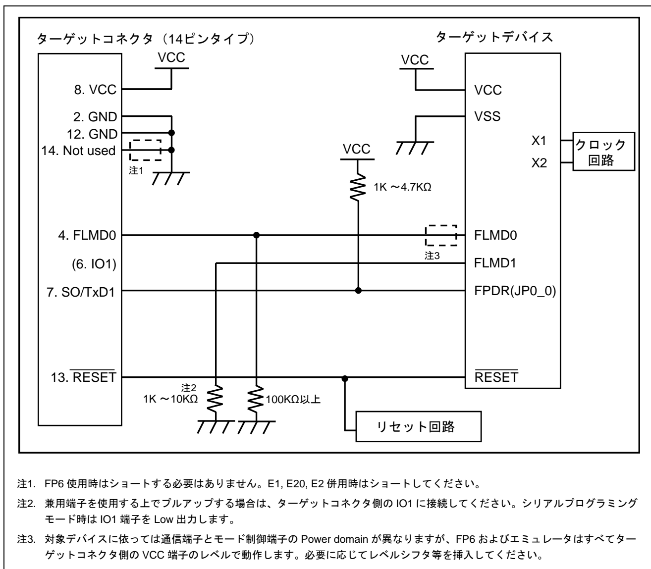
図 3.8 1 wire UART (RH850ファミリ) の回路例 (RH850/F1xの回路例)
