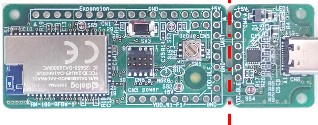
モジュール基板
