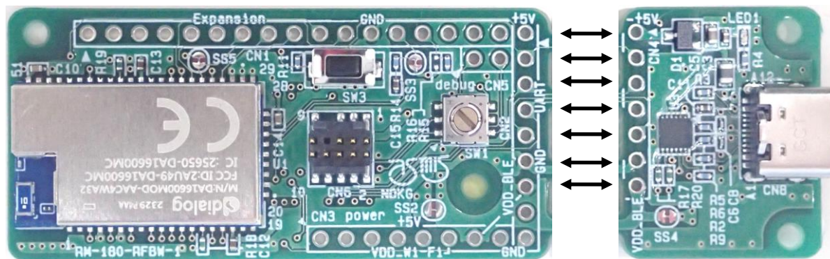
図 3-3 基板分割
